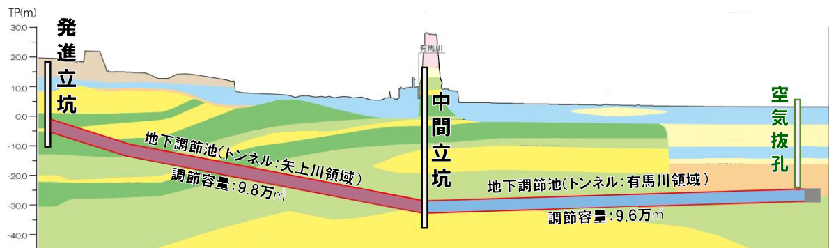
縦断面図
