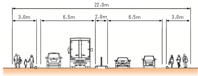
標準横断図
