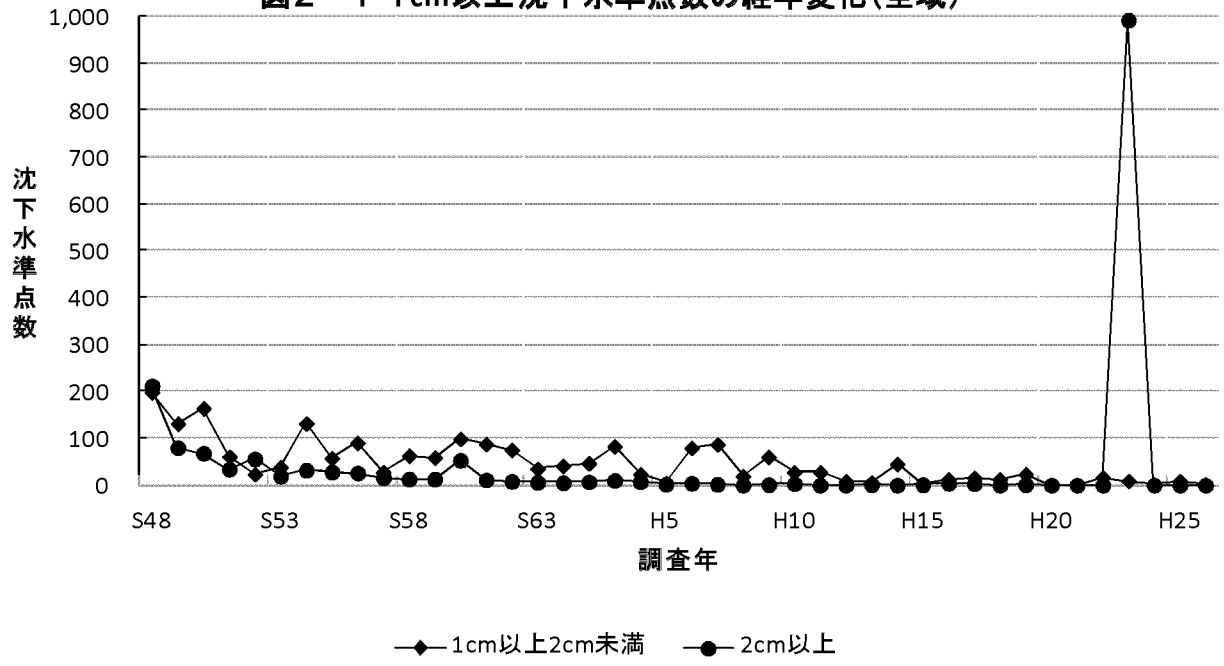
図2-1 1cm以上沈下水準点数の経年変化(全域)
