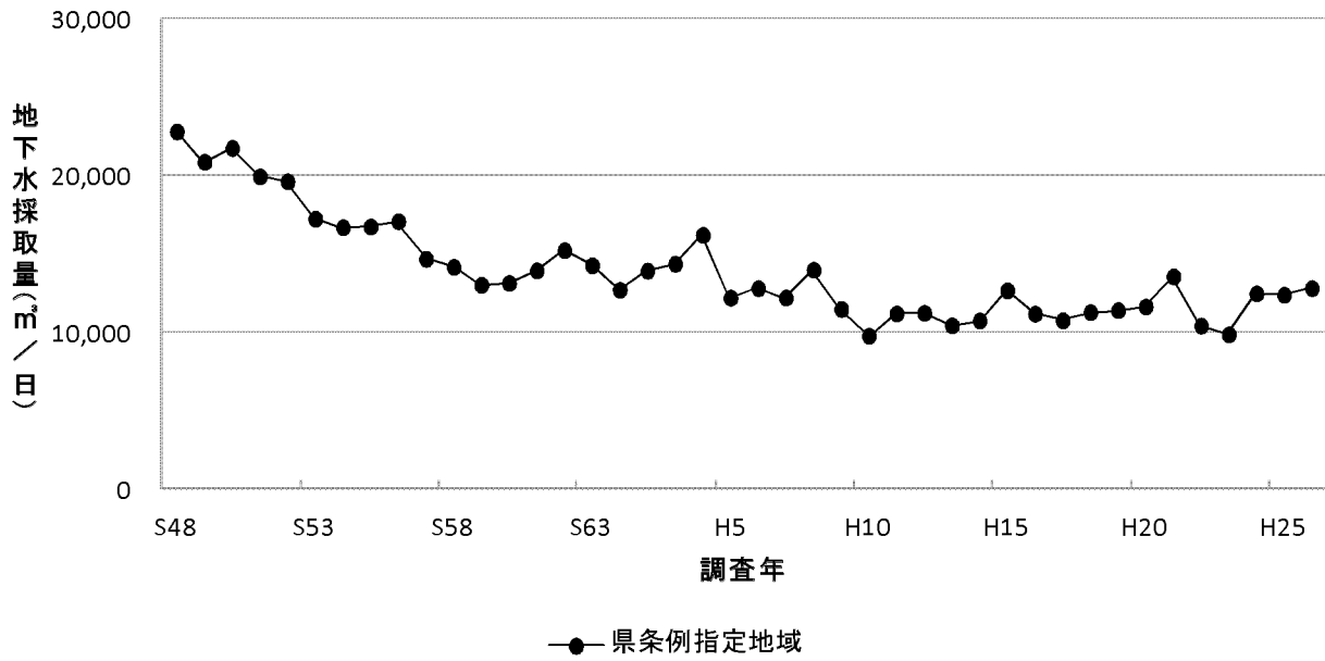
図1-7 地下水採取量の経年変化(寒川町)
