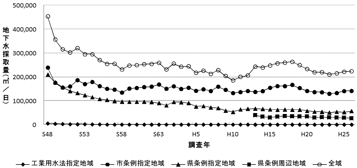
図1-10 地下水採取量の経年変化(全域)
