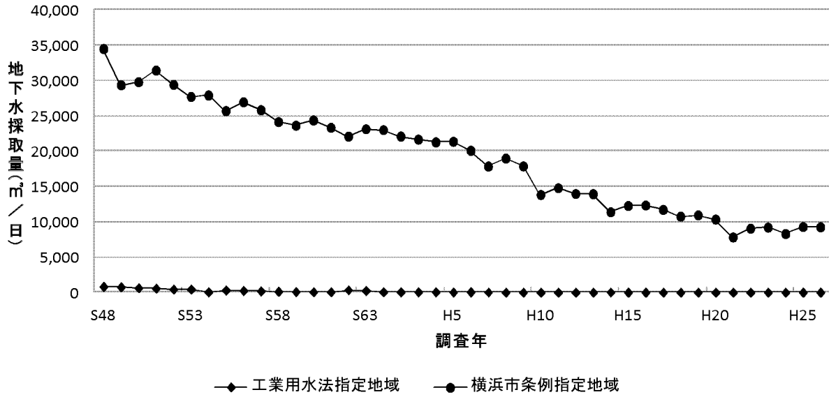
図1-1 地下水採取量の経年変化(横浜市)
