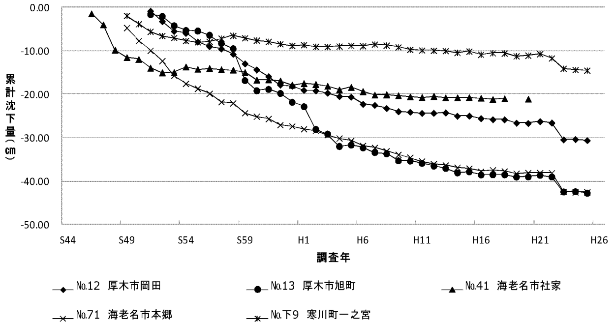
図5-2 主要水準点の沈下状況の経年変化 県央・湘南地域(2)
