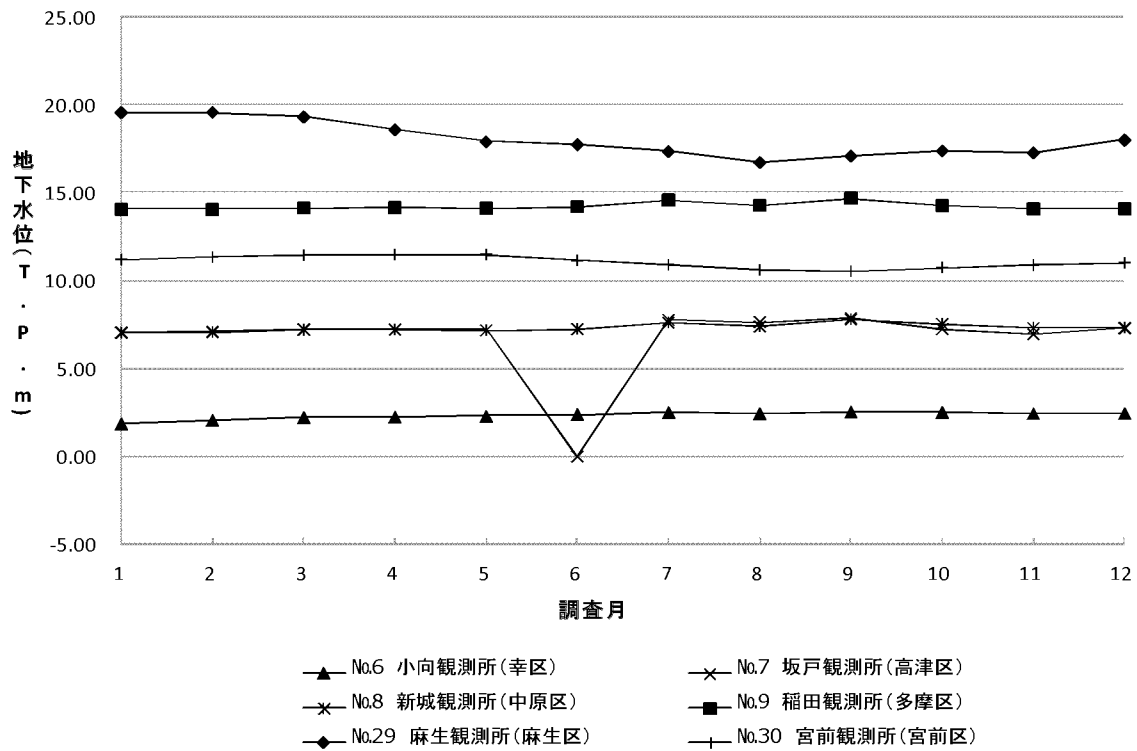
図7-8 平成27年地下水位の経月変化(川崎市幸、高津、中原、多摩、麻生、宮前区)
