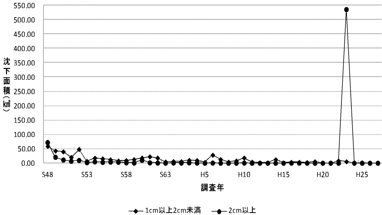
図2-2 1cm以上沈下面積の経年変化(全域)
