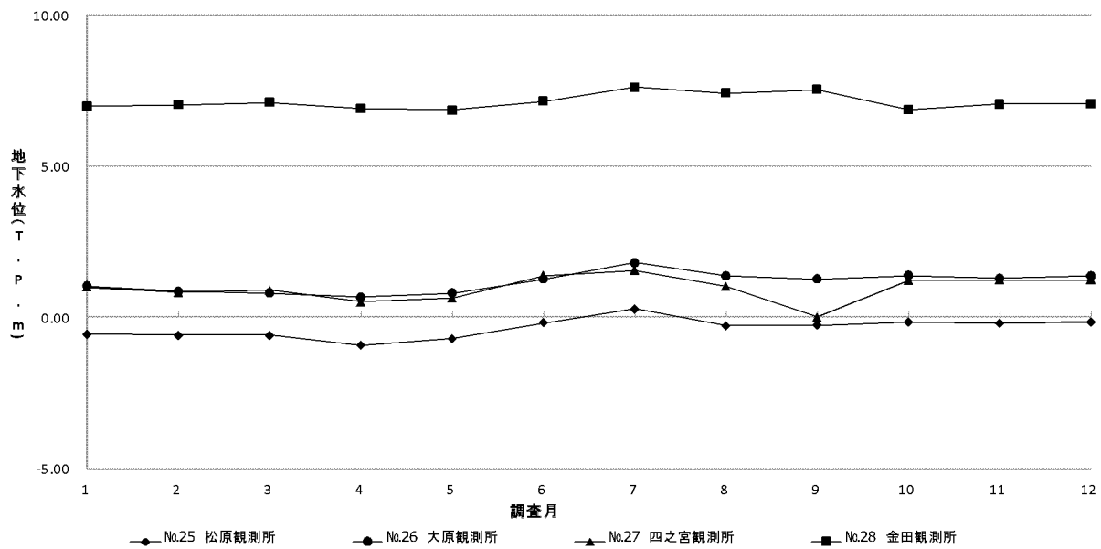
図7-9 平成27年地下水位の経月変化(平塚市)
