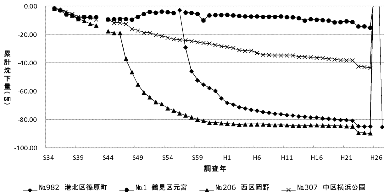
図3-1 主要水準点の沈下状況の経年変化 横浜地域(1)
