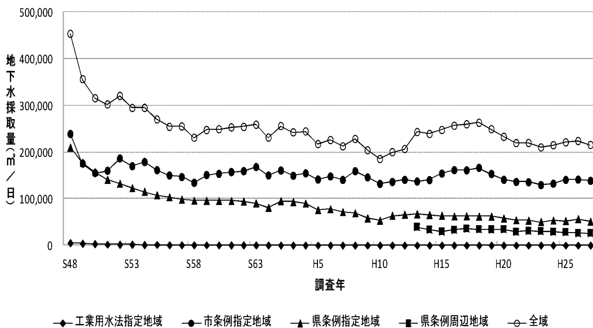
図1-10 地下水採取量の経年変化(全域)
