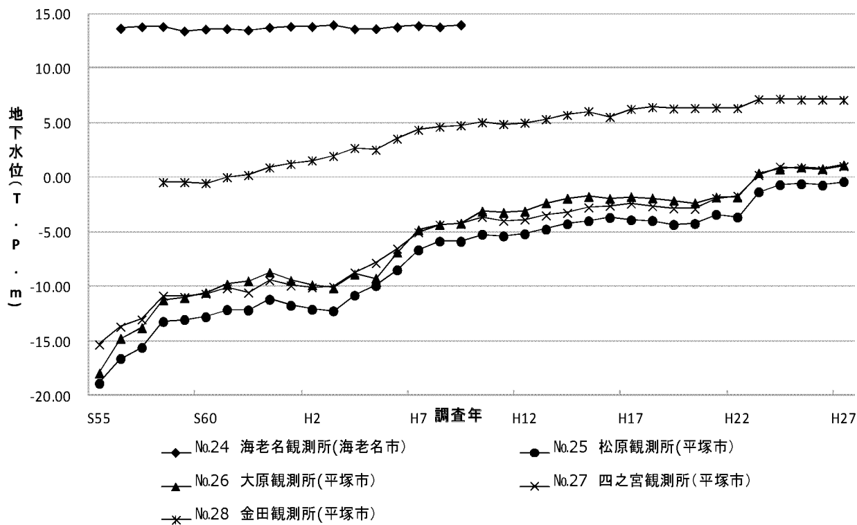
図7-6 地下水位の経年変化(平塚市、海老名市、寒川町)
