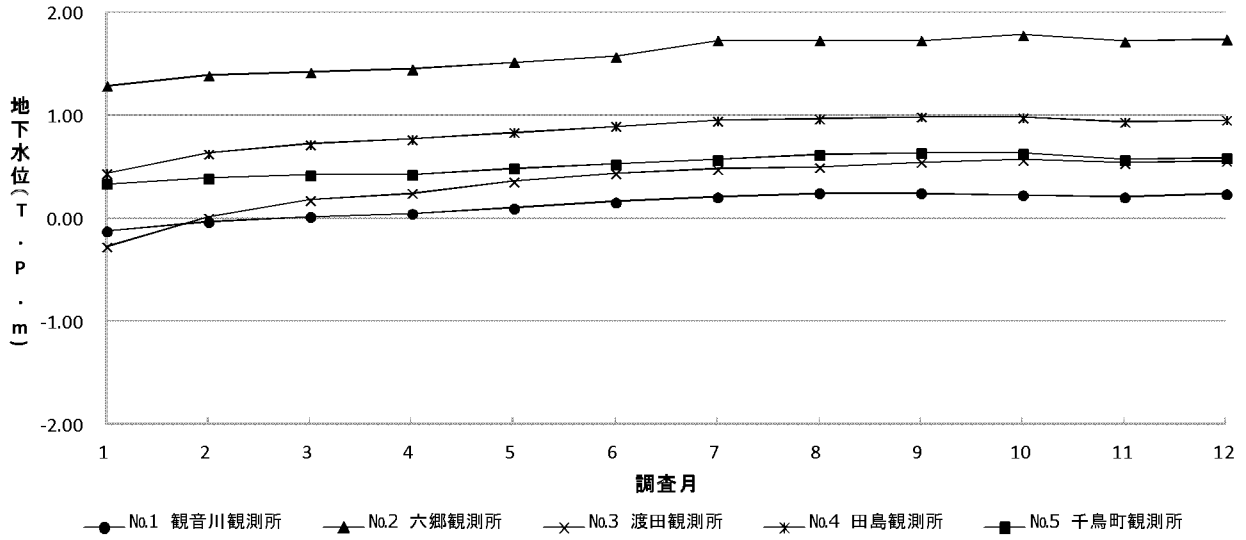
図7-7 平成27年地下水位の経月変化(川崎市川崎区)
