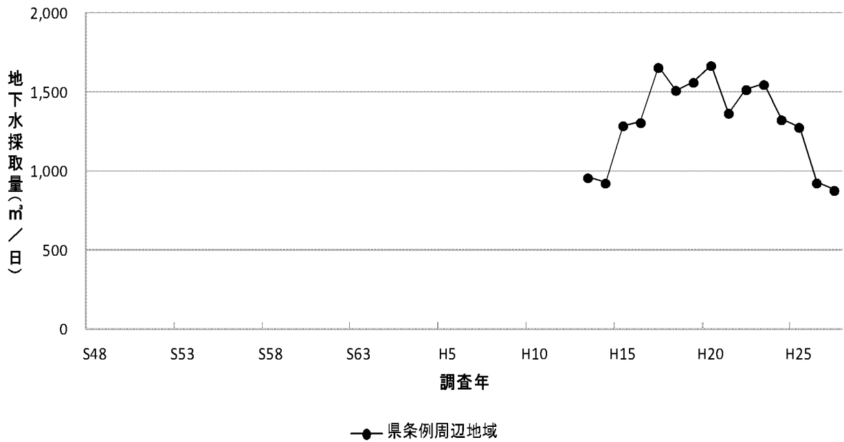
図1-8 地下水採取量の経年変化(鎌倉市)
