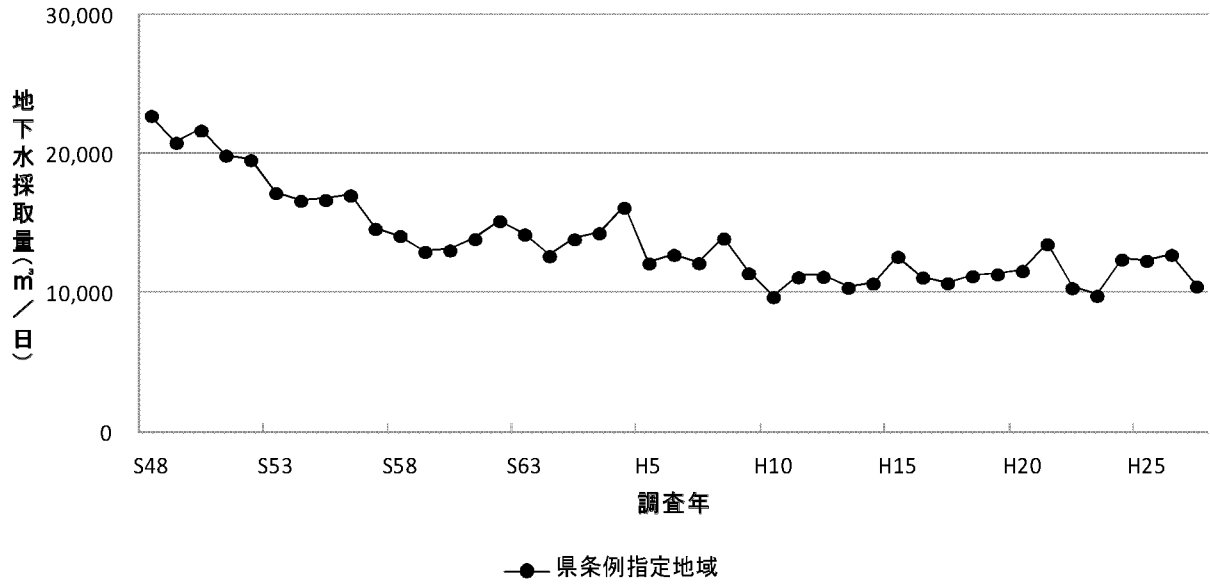
図1-7 地下水採取量の経年変化(寒川町)
