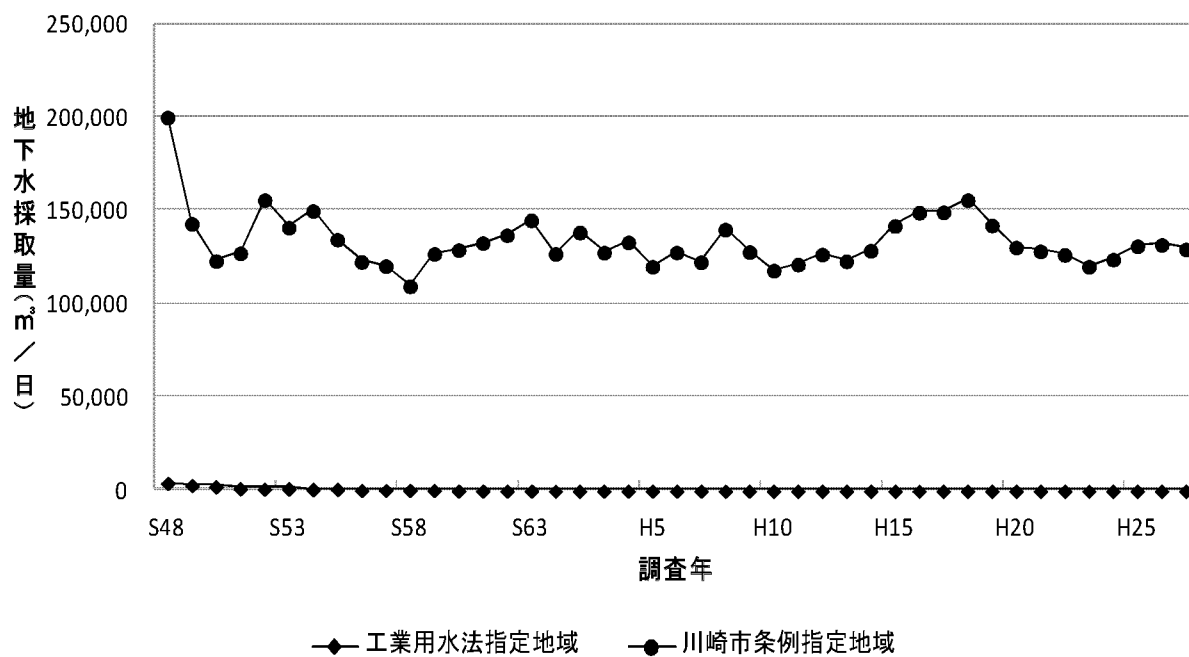
図1-2 地下水採取量の経年変化(川崎市)
