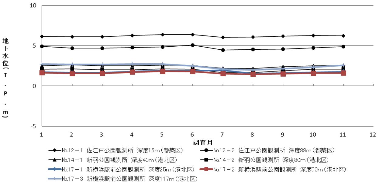
図5-3 令和5年地下水位の経月変化(横浜市都筑区、港北区)
