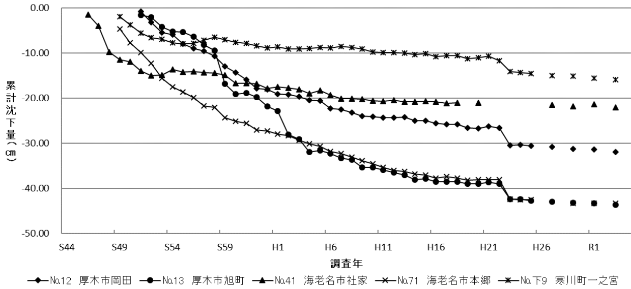
図3-5 主要水準点の沈下状況の経年変化 県央・湘南地域(2)
