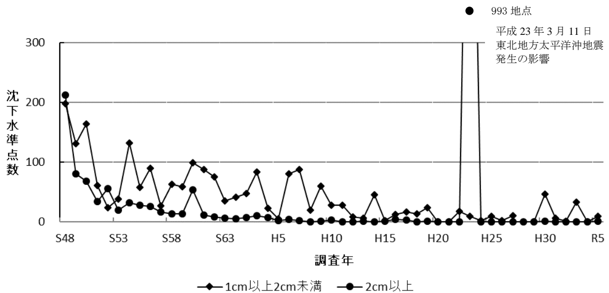
図2 1cm以上沈下水準点数の経年変化(全域)
