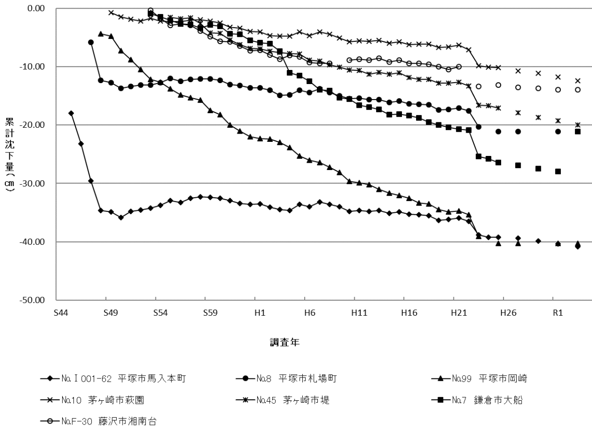
図3-4 主要水準点の沈下状況の経年変化 県央・湘南地域(1)
