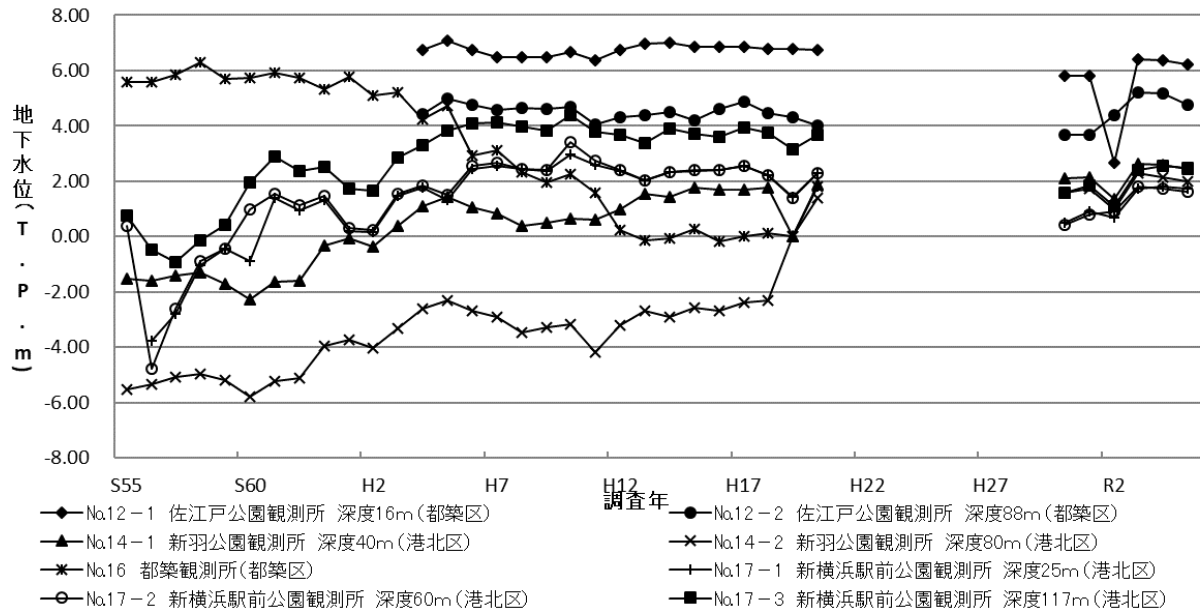
図6-3 地下水位の経年変化(横浜市都筑区、港北区)
