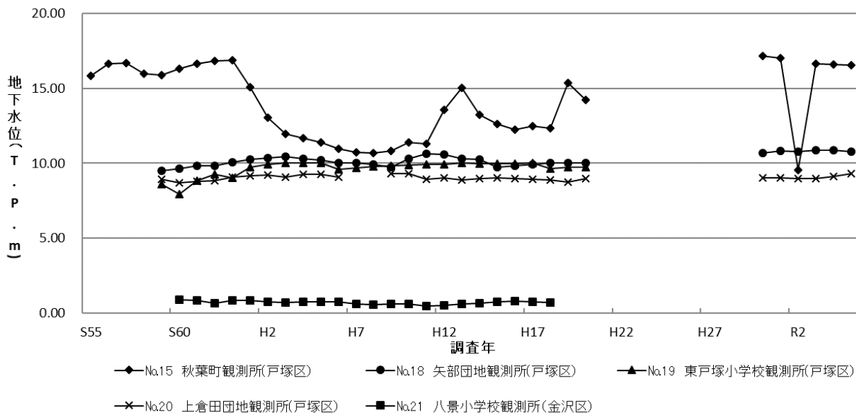
図6-5 地下水位の経年変化(横浜市戸塚区、金沢区)
