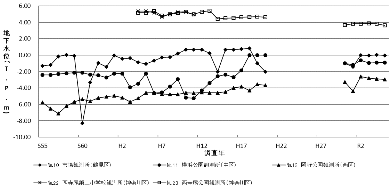
図6-4 地下水位の経年変化(横浜市鶴見区、神奈川区、西区、中区)
