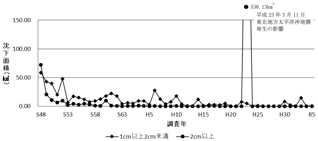
図1 1cm以上沈下面積の経年変化(全域)
