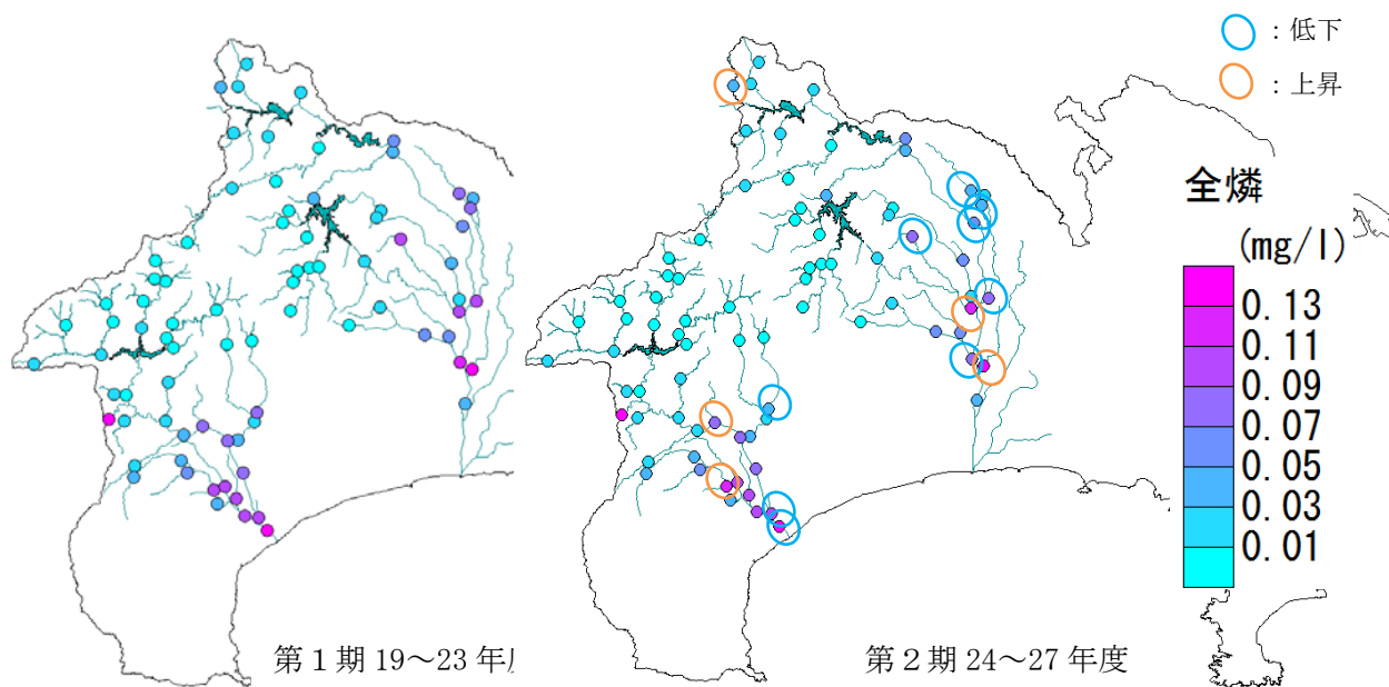
図9 全燐の経年変化
