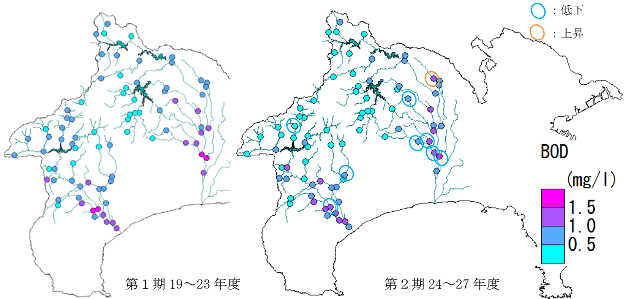
図 7 BOD の経年変化
