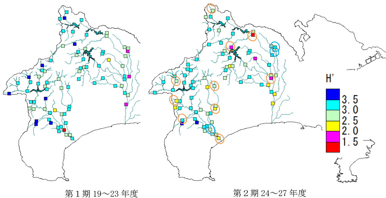
図4 多様度指数の経年変化
