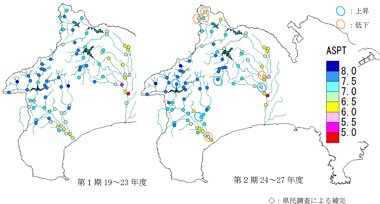
図 3 平均スコア値の経年変化
