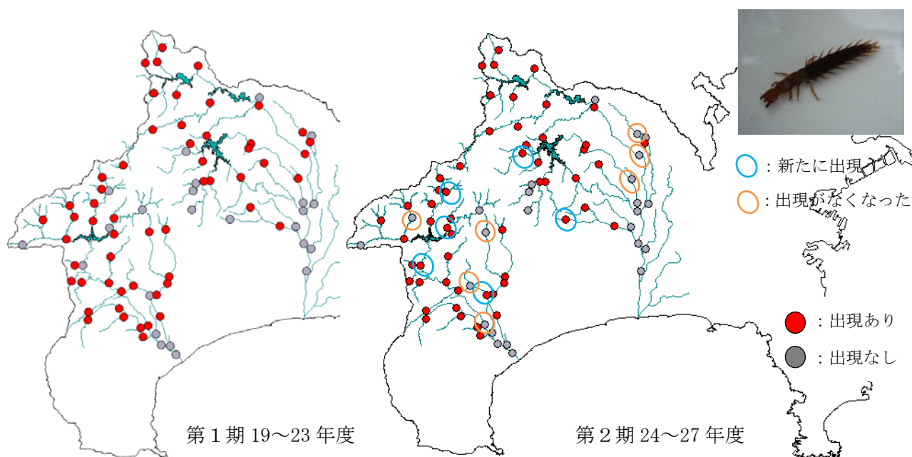
図6 ヘビトンボ出現状況の経年変化
