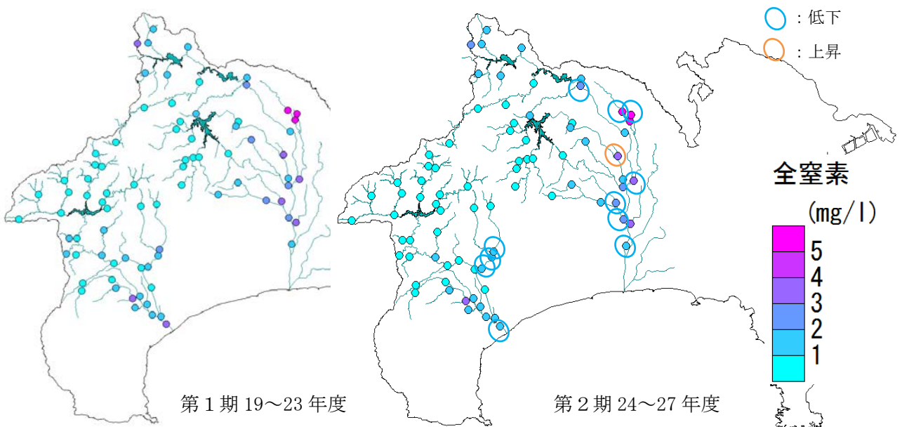
図 8 全窒素の経年変化
