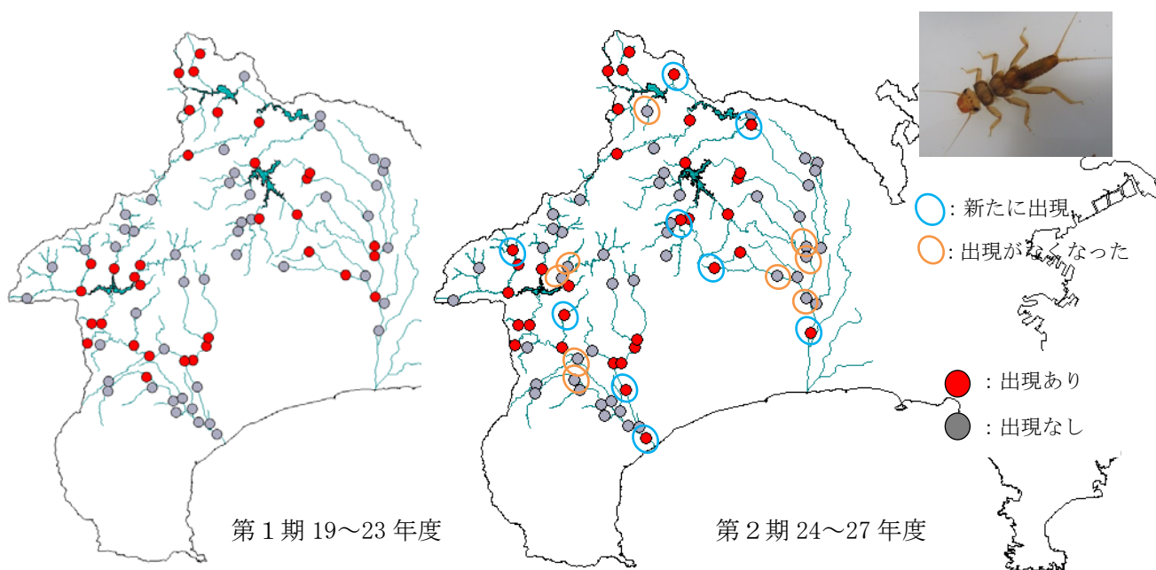
図5 カミムラカワゲラ出現状況の経年変化
