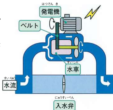
小水力発電のしくみ (例)
