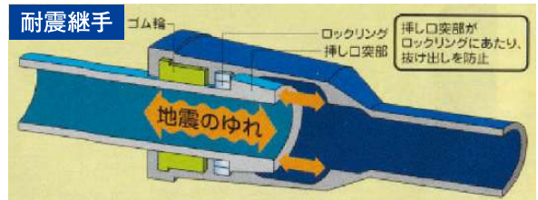
つなぎ目がはずれにくい丈夫な水道管 (耐震継手管)
