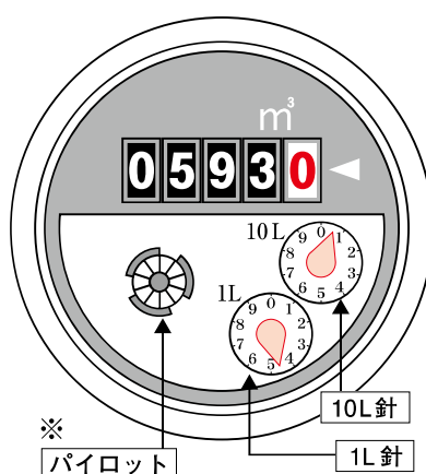
標準的な 水道メータ
