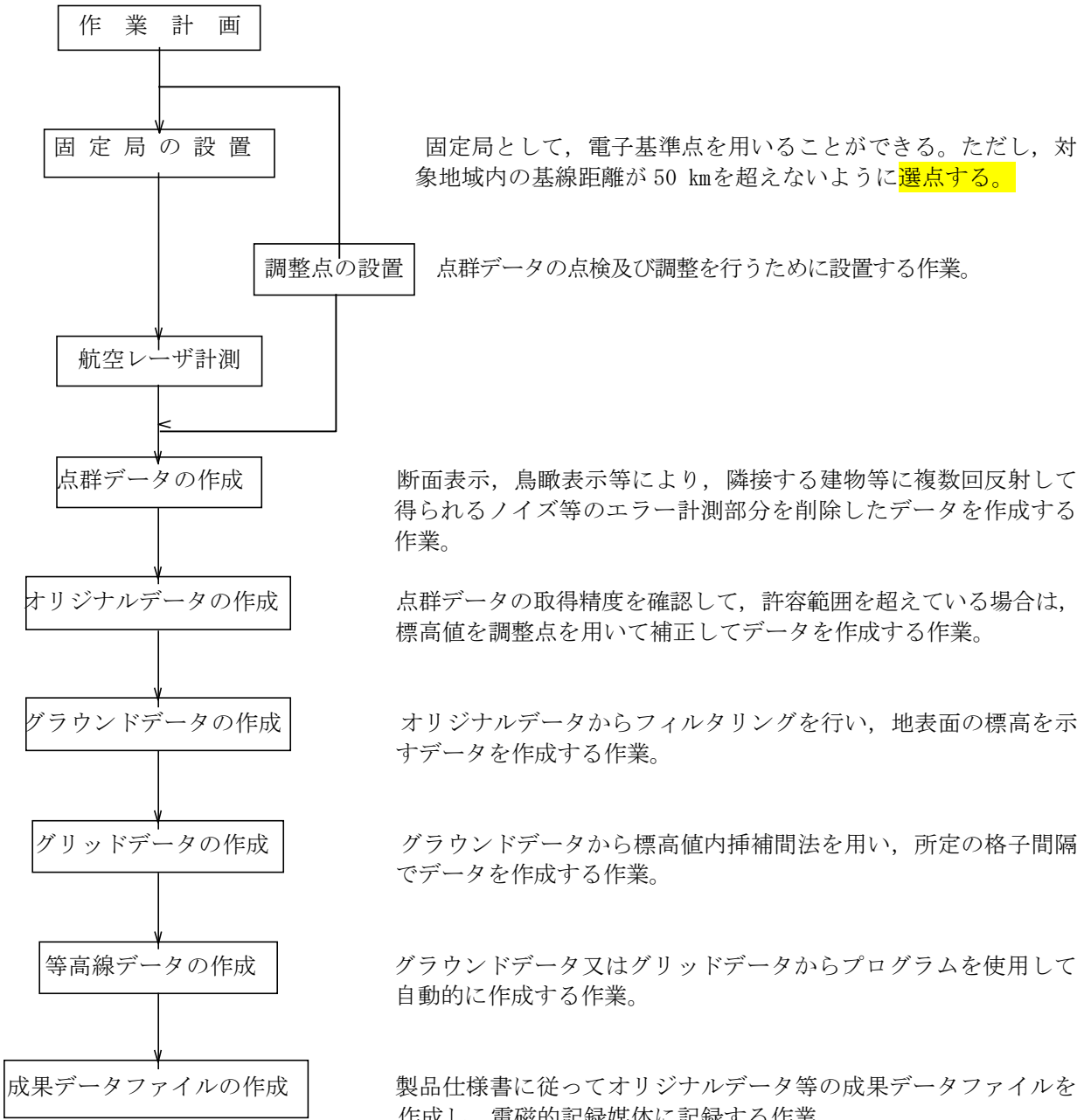
図 2－6－1 航空レーザ測量フローチャート
