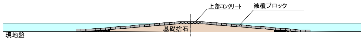
C断面
