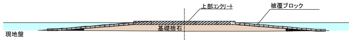
B断面
