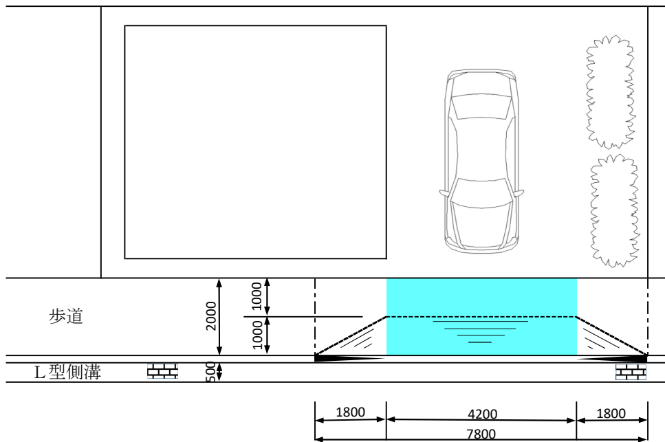
(計画平面図)
