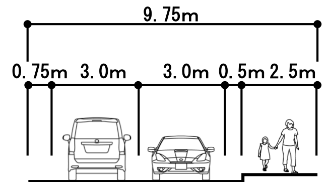
○バイパス区間の横断面図
