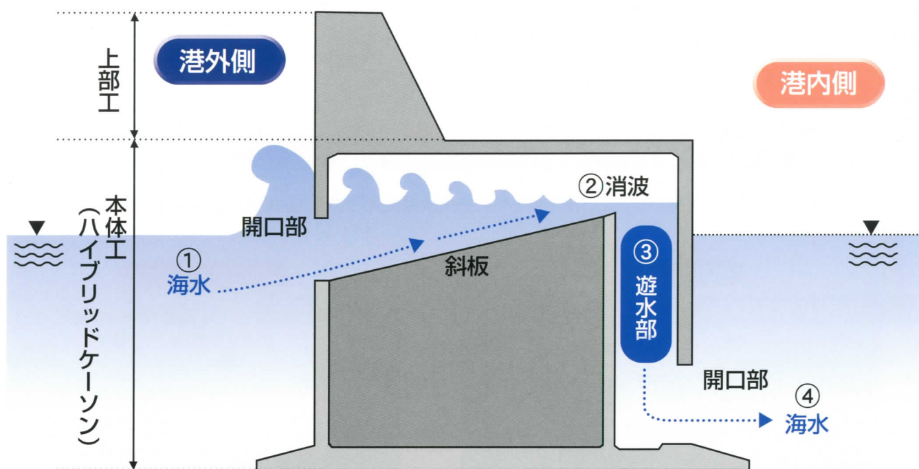
海水交換型防波堤の内部
