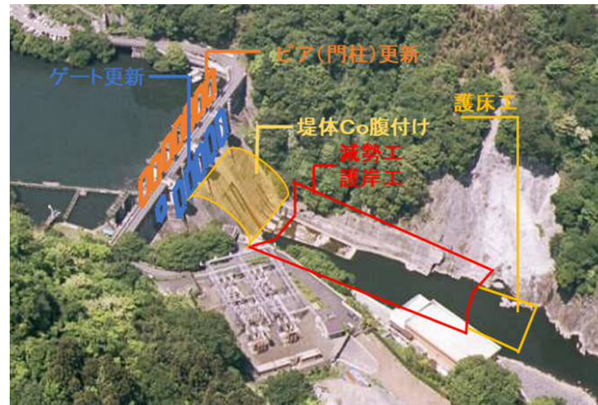
相模ダムリニューアル事業図
