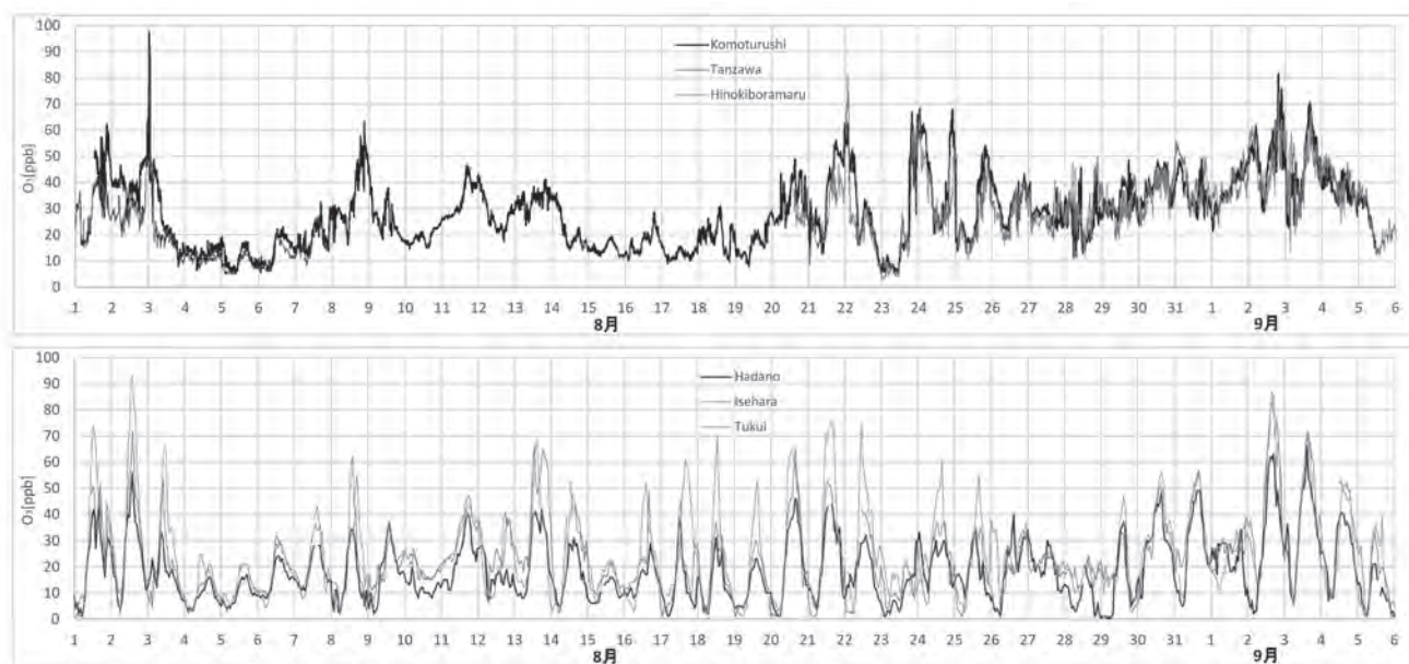
図2-3 2014年8月1日から9月5日の丹沢山地オゾン濃度（菰釣山、丹沢山、檜洞丸＝10分値、上）と周辺一般局（秦野、伊勢原、津久井＝1時間値、下）におけるオゾン濃度
