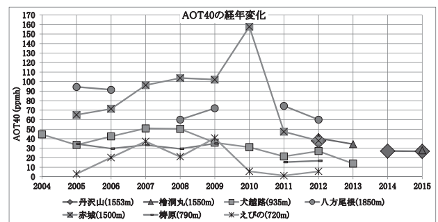
図 2-8 丹沢山地と国設酸性雨局の AOT40 の経年変化
