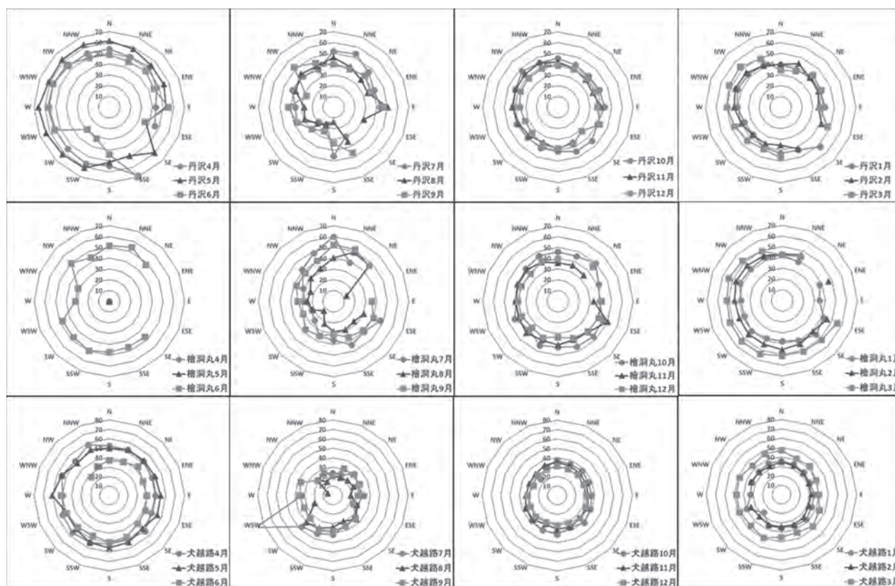
図 2-9 2012 年度丹沢山地測定局の風向別平均オゾン濃度
