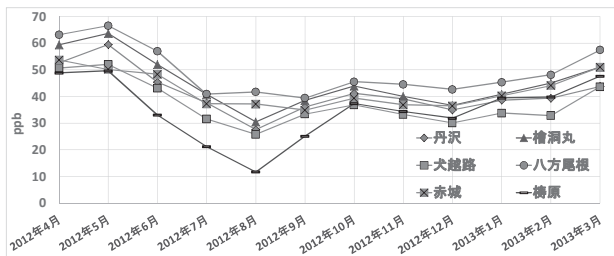
図 2-7 丹沢山地と国設酸性雨局の 2012 年度月平均値
