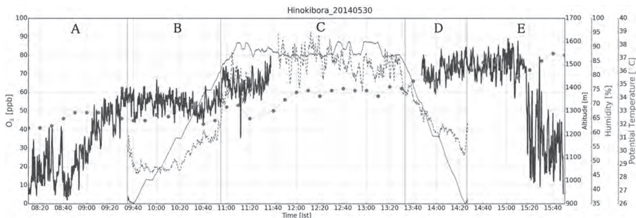
図 3-3 2014 年 5 月 30 日檜洞丸移動観測結果 (太実線:2B202 オゾン、破線:温位、丸:檜洞丸オゾン 10 分値、細実線:標高)
