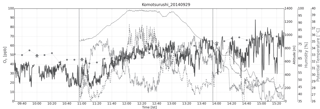
図 3-5 2014 年 9 月 29 日菰釣山移動観測結果 (太実線: 2B202 オゾン、破線: 温位、点線: 相対湿度、丸: 檜洞丸 10 分値、星: 菰越路オゾン 1 時間値、細実線: 標高)
