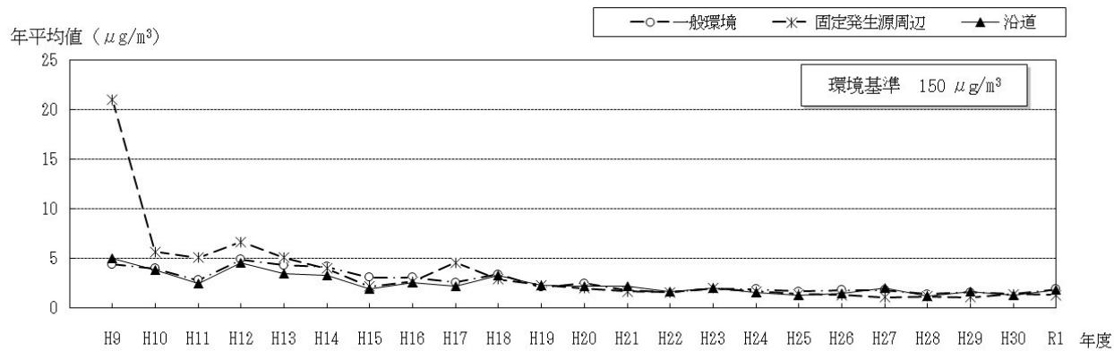
図 8-1-5 ジクロロメタンの地域分類ごとの年平均値の経年推移
