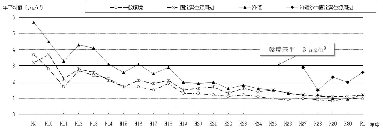
図 8-1-2 ベンゼンの地域分類ごとの年平均値の経年推移
