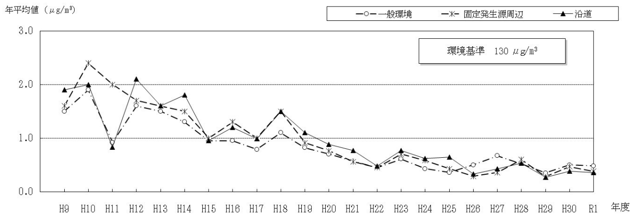
図 8-1-3 トリクロロエチレンの地域分類ごとの年平均値の経年推移
