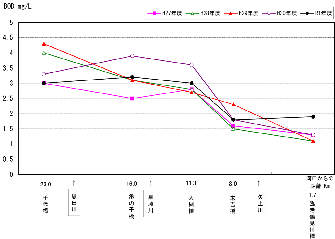
図2-2 鶴見川におけるBOD縦断変化図
