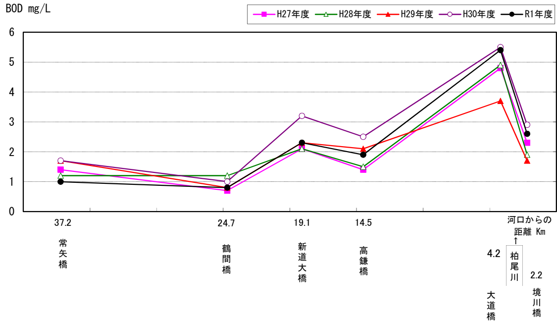
図2-3 境川におけるBOD縦断変化図
