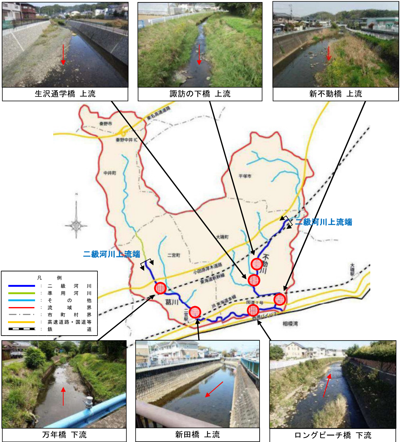
図 1-8 河道現況
