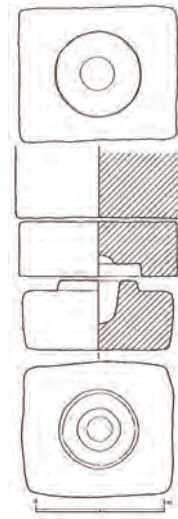
静岡県沼津市清水柳北1号墳石櫃 S=1/8
