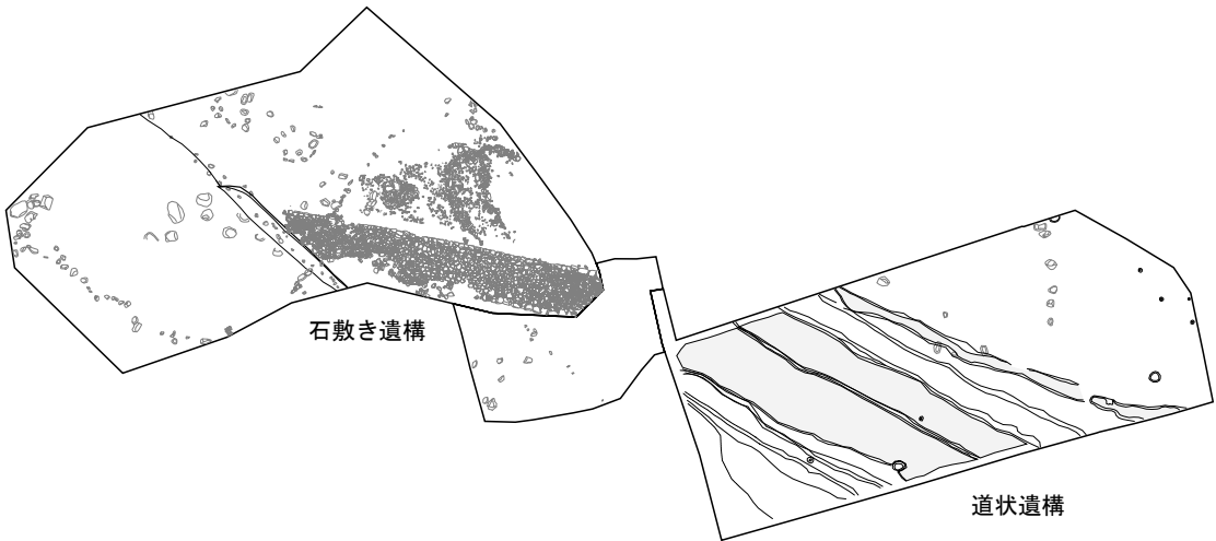
第5図 上粕屋・子易2遺跡石敷き遺構
