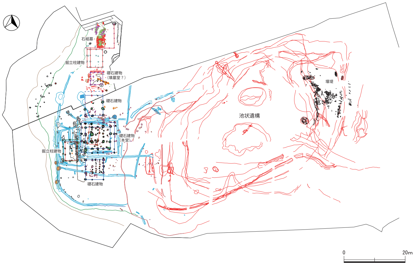
第7図 子易・中川原遺跡中世寺院図
