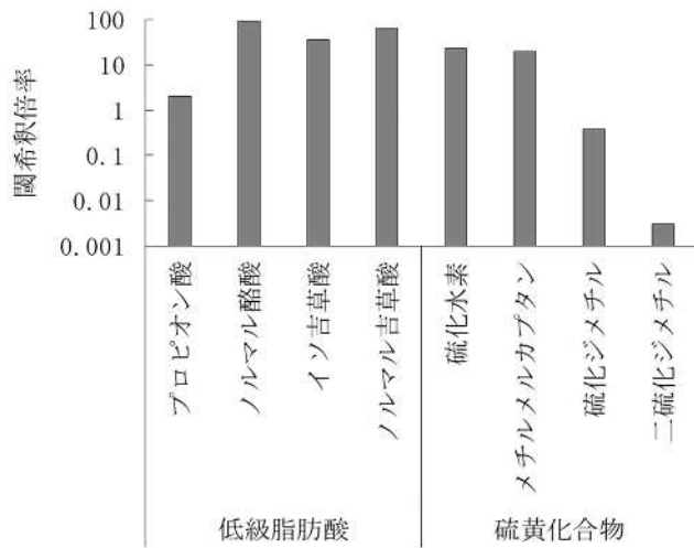
図1 豚舎排気中の悪臭物質濃度
