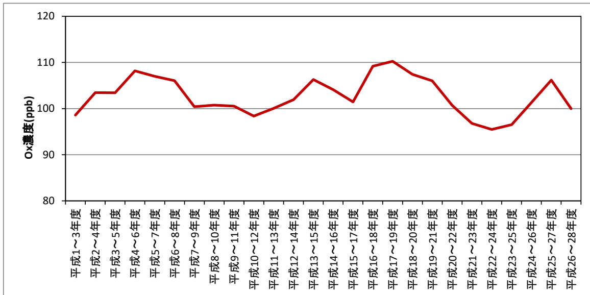
(1) 一般環境大気測定局における新指標の県内最高値の経年変化
