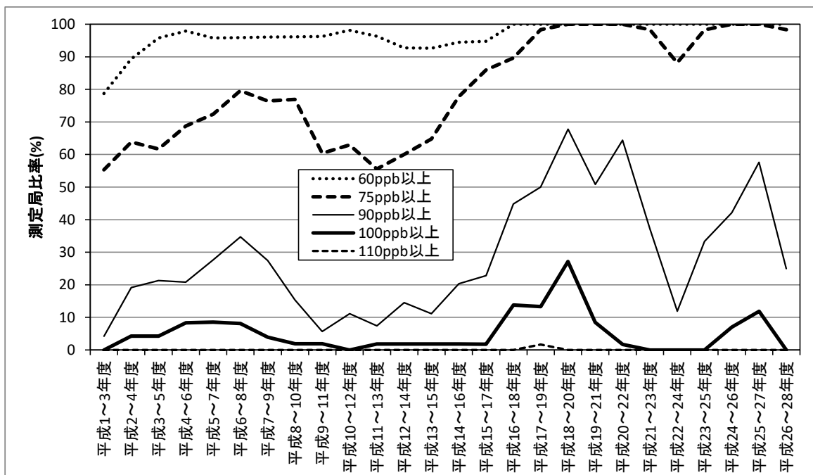
(2) 一般環境大気測定局における新指標が一定濃度以上となる局数の経年変化
