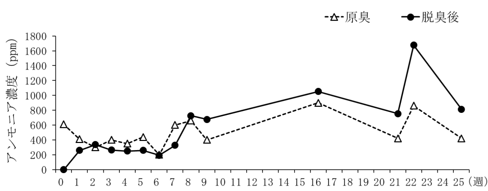
図1 脱臭前後のアンモニア濃度および除去率の推移
