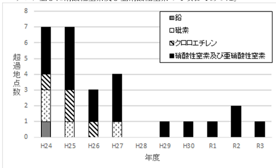
図5 定点調査における項目別の環境基準超過地点数の経年変化
