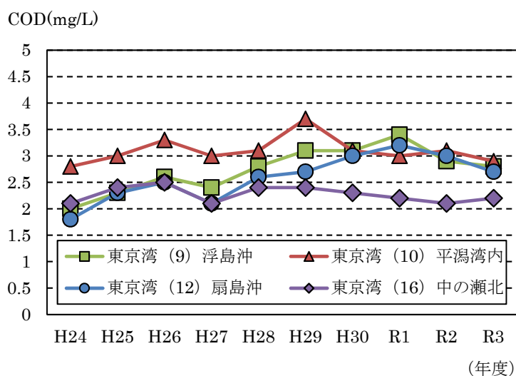
図3 海域の環境基準非達成地点におけるCODの年間平均値の推移
